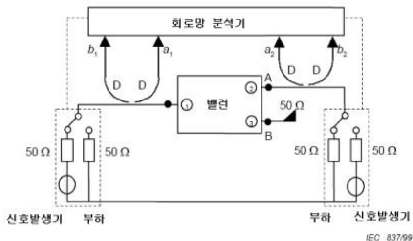
그림 B.2. 신호발생기와 부하를 서로 바꾸었을 때(이 그림에서, 양쪽의 스위치를 반대위치로 전환함으로써), S_{11} 과 S_{12} , 및 S_{22} 와 S_{21} 의 측정도
